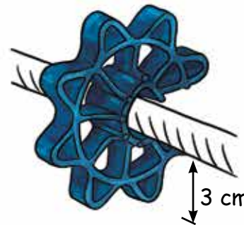
separador industrial
